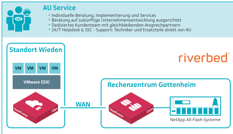
Infrastrukturskizze SensoPart
