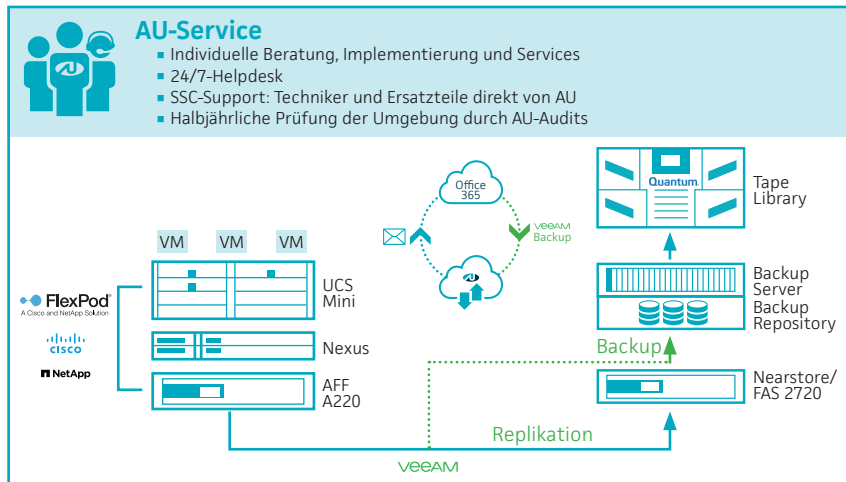
Infrastruktursskizze PTW
